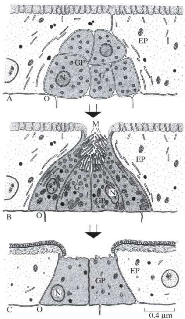
Рис. 3. Схема формирования и строения половой поры у I. variabilis . Обозначения: EP – эпителиальная клетка, G – гранулы, GP – клетки генитальной поры, M – микровилли, N – ядро, O – ооцит. А, В, С – последовательные стадии формирования половой поры.
